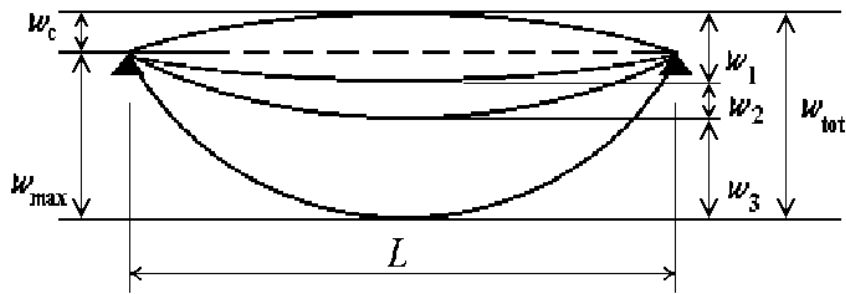
Фигура NA.7.1 Определяне на вертикални премествания
